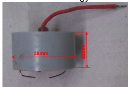
Nagyfesz tekercsek
