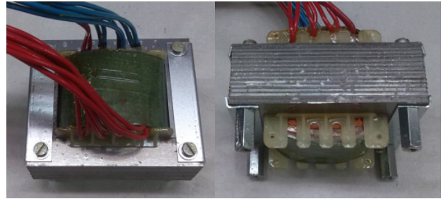
Nagyfesz tekercsek
